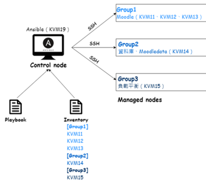
ansible 架構原理及工作流程
